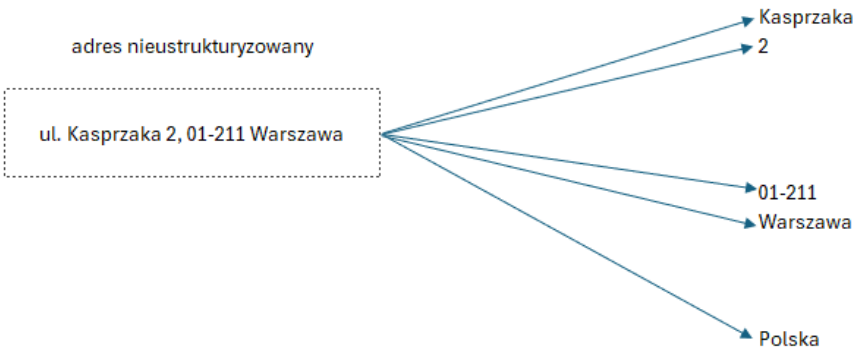
Mapowanie adresu pocztowego do formuły adresu hybrydowego (częściowo ustrukturyzowanego)
